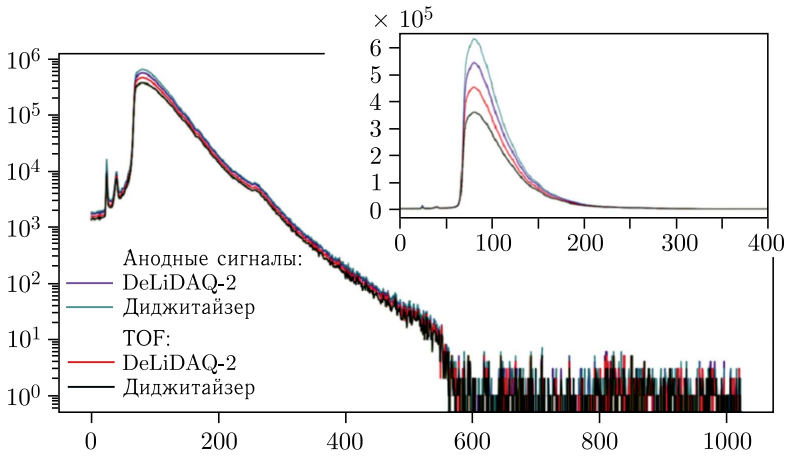
Рис. 4. Прямой пучок. DeLiDAQ-2 и диджитайзер. Графики анодных сигналов и TOF в логарифмическом и линейном (справа сверху) масштабах
