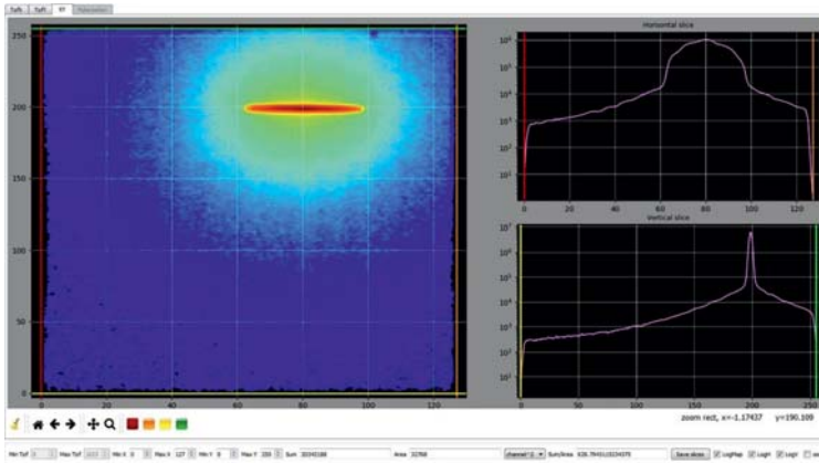
Рис. 2. Прямой пучок, диджитайзер
