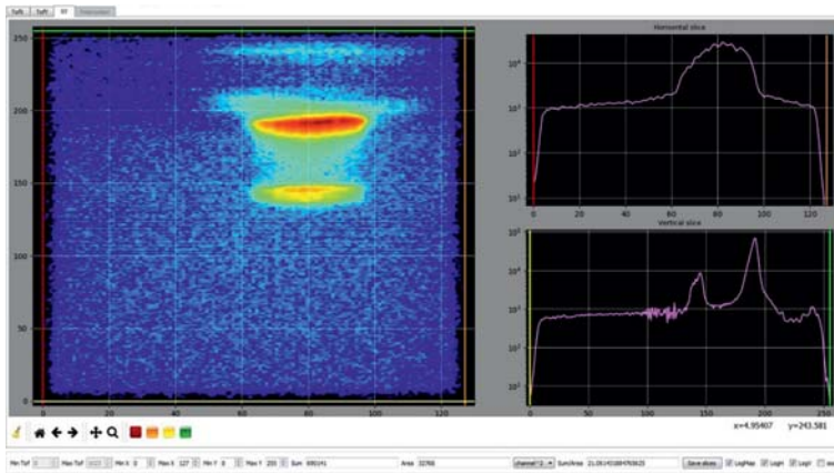
Рис. 6. Образец Si/SiO 2 , DeLiDAQ-2
