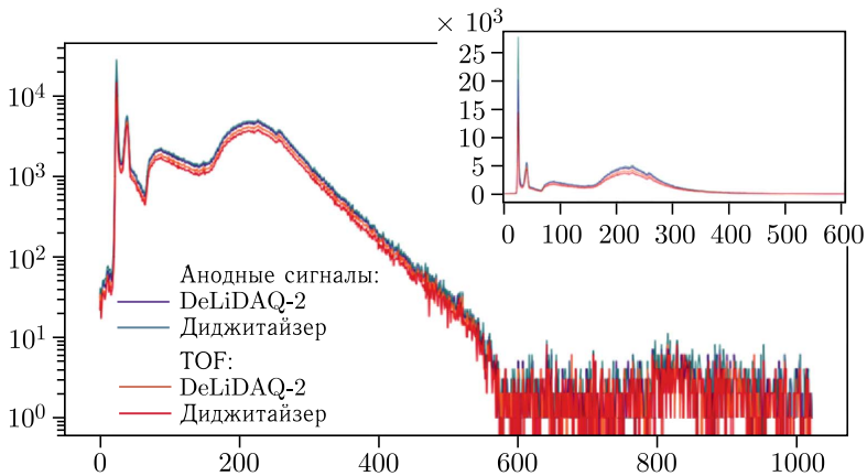
Рис. 7. Образец Si/SiO 2 , DeLiDAQ-2 и диджитайзер. Графики анодных сигналов и TOF в логарифмическом и линейном (справа сверху) масштабах
