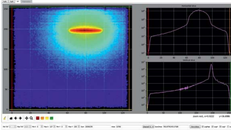
Рис. 3. Прямой пучок, DeLiDAQ-2
