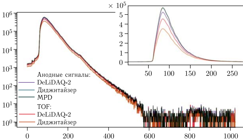
Рис. 8. Прямой пучок. DeLiDAQ-2 и диджитайзер. TOF и анодные сигналы с добавлением MPD
