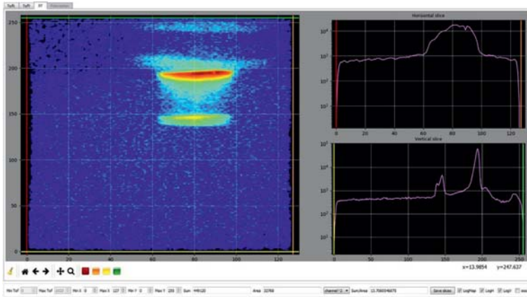
Рис. 5. Образец Si/SiO 2 , диджитайзер
