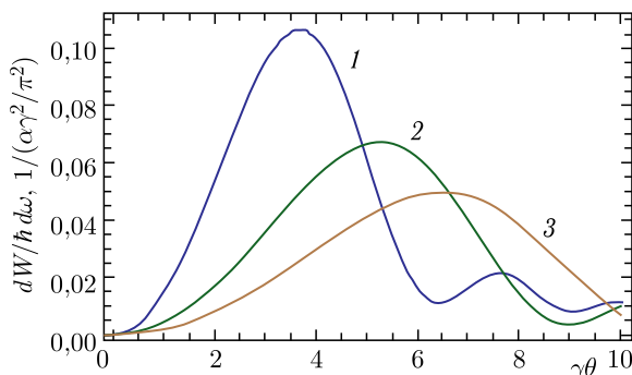
Рис. 8. Угловые распределения переходного излучения с различной длиной волны для фиксированного расстояния между мишенью и апертурой D = 150 мм при \gamma = 100 : кривая 1 — \lambda = 0,3 мм; кривая 2 — \lambda = 0,6 мм; кривая 3 — \lambda = 0,9 мм
