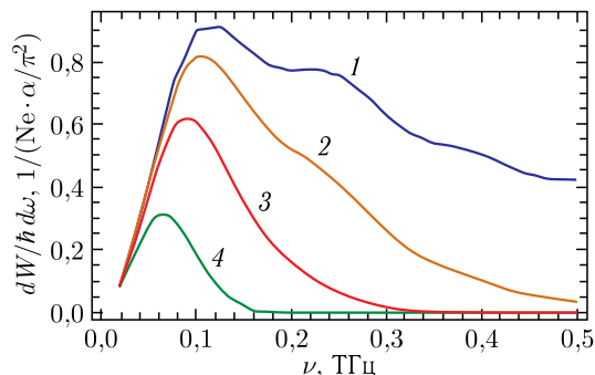
Рис. 11. То же самое, что и на рис. 10, для угла поворота мишени \psi = 48,5^\circ : кривая 1 — спектр некогогерентного переходного излучения; кривая 2 — длина сгустка \sigma_z = 0,15 мм; кривая 3 — \sigma_z = 0,3 мм; кривая 4 — \sigma_z = 0,6 мм
