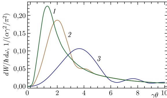
Рис. 7. Угловые распределения переходного излучения с фиксированной длиной волны \lambda = 0,3 мм на различных расстояниях от мишени в предволновой зоне для \gamma = 100 : кривая 1 — D = 1500 мм; кривая 2 — D = 500 мм; кривая 3 — D = 150 мм
