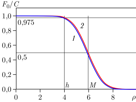
Рис. 1. Функция распределения с плоской вершиной (монопольная мода)
