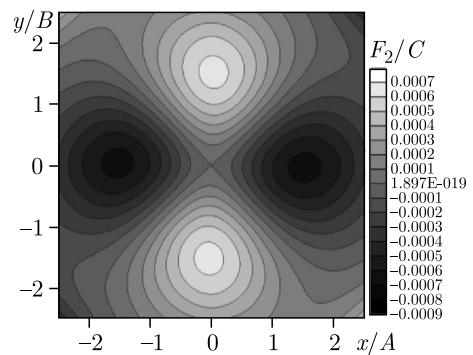
Рис. 4. Линии уровня квадрупольной моды ( k = 2 ) вблизи оси
