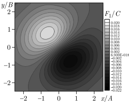
Рис. 3. Линии уровня дипольной моды ( k = 1 ) вблизи оси
