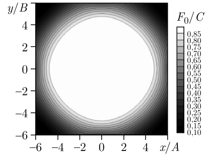
Рис. 2. Линии уровня монопольной моды ( k = 0 )
