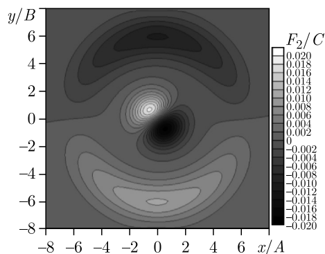
Рис. 5. Линии уровня дипольной моды ( k = 1 ) с учетом периферии
