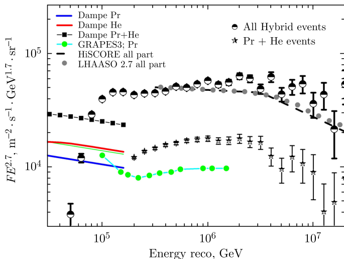
Рис. 3 (цветной в электронной версии). Темные кружки — восстановленный спектр всех частиц из гибридных событий; темные звездочки (условно Pr + He) — спектр легкой компоненты, восстановленный из событий с \text{width} < \text{widthCut}(\text{size}) ; красные и синие линии — прямые измерения спутникового эксперимента Dampe протонов и гелия [8]; черная штриховая линия — спектр всех частиц, полученный только по данным в работе в HiSCORE [2]; серые точки — в эксперименте LHAASO [7]; зеленые точки — оценка спектра протонов в эксперименте GRAPES3 [9]
