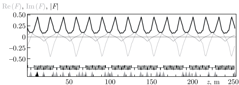
Рис. 2. Функция отклика дейтронов для энергии 270 МэВ/нуклон
