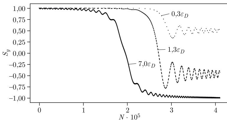
Рис. 4. Изменение вертикальной проекции спина дейтрона при пересечении индуцированного резонанса для трех значений амплитуд бетатронных колебаний, соответствующих быстрому пересечению (пунктирная кривая, \varepsilon_y = 0,3\varepsilon_D ), промежуточному пересечению (штриховая кривая, \varepsilon_y = 1,3\varepsilon_D ) и медленному пересечению (сплошная кривая, \varepsilon_y = 7,0\varepsilon_D )
