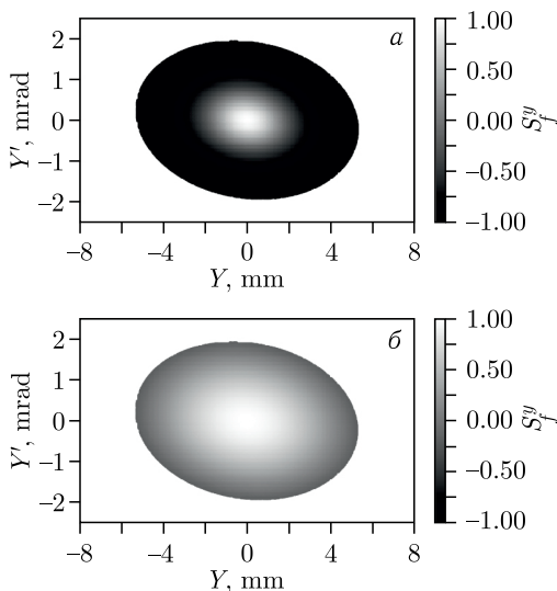
Рис. 1 (цветной в электронной версии). Профиль поляризации для частиц при медленном (а) и промежуточном (б) пересечениях резонанса
