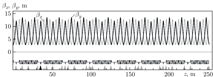
Рис. 3. Бета-функции дейтронов в нуклотроне
